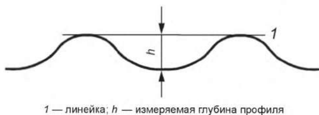
Рисунок А.1 — Измерение глубины профиля h для черепицы с волнистым профилем
