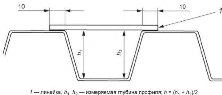
Рисунок А.2 — Измерение глубины профиля h для металлочерепицы с трапецевидным профилем
