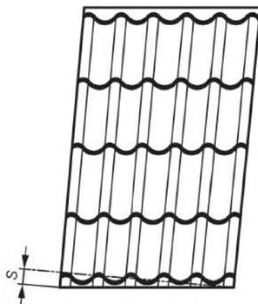
Рисунок 7 — Косина реза
