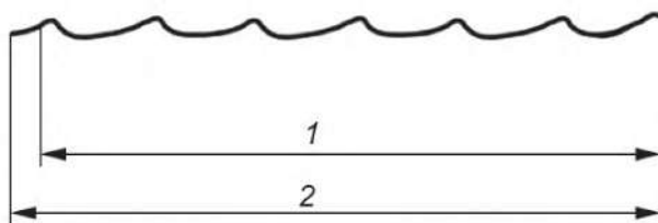
Рисунок 5 — Полезная и полная ширина изделия
